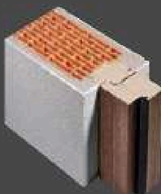
RAHMENSTOCK RS in der Laibung mit Blindstock montiert
