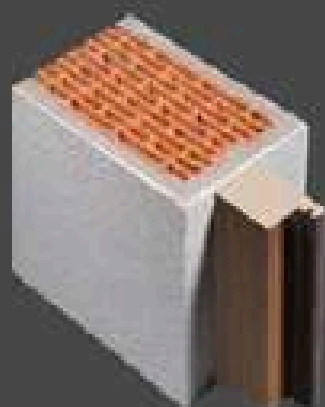
BLENDRAHMEN BW 40005 in der Laibung montiert (ke labige Position)
