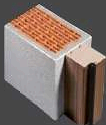
RAHMENSTOCK RS in der Laibung montiert (ke labige Position)
